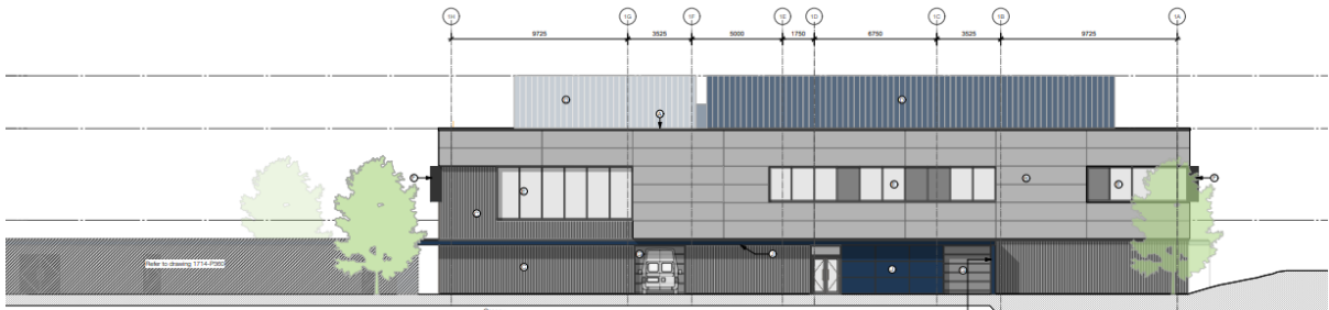
01 Elevation
